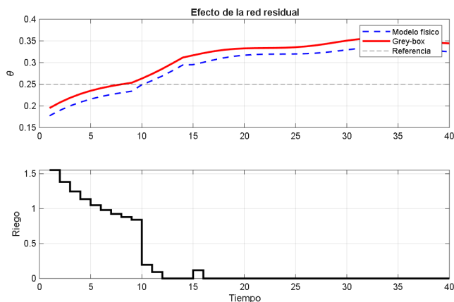
Figura 13. Comparación entre el modelo físico y el esquema Grey-Box dentro del MPC.
